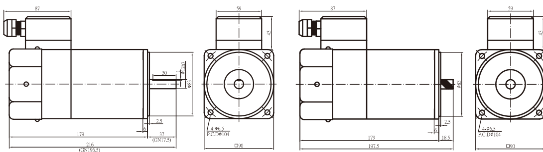
60W/60W-GX外型圖
