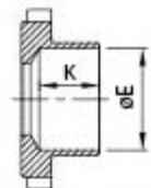
差込み溶接
