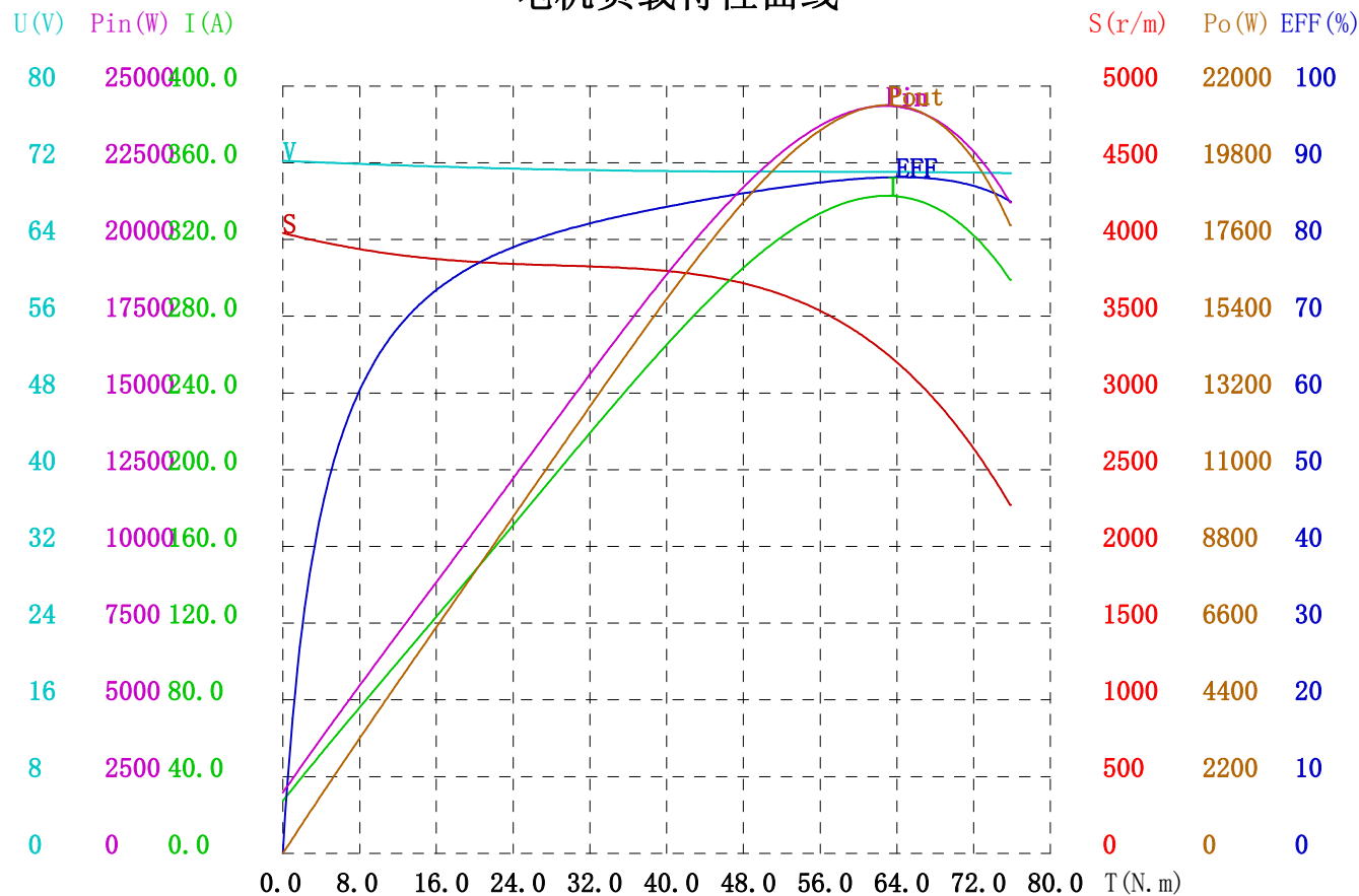
电机负载特性曲线
