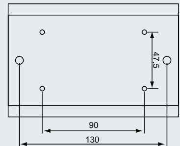
CSR-A03 (For CTR10A-120A)
