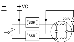
5、Motor positive and reverse Application Circuit 电机正反转应用电路
