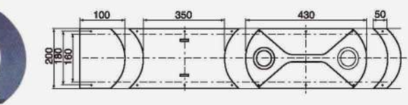
B 豪华出风口 Wind Outlet 外形尺寸(Dimension): 430 × 200 开孔尺寸(Dimension): 430 × 160
