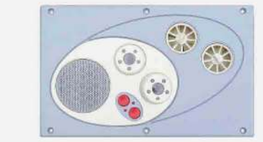
CD25-026 出风口 Wind Outlet 外形尺寸(Dimension): 350 × 220 开孔尺寸(Dimension): 320 × 180
