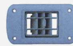
CD22-001 单出风口 Whirl single wind outlet 外形尺寸(Outline size): 127 x 73 开孔尺寸(Hole size): 65 x 54
