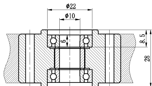
安装部分剖面图
