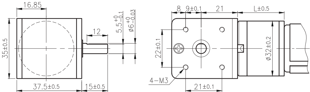
外形尺寸/ Appearance Size
