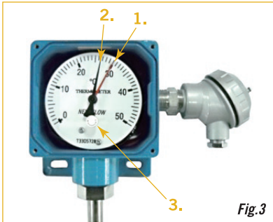
Fig.3: 1. 設定點紅色指針(Alarm用)。 功能: 指示Alarm設定值用。 Setpoint red indicator (for alarm). Function: Alarm setpoint indication. 2. 黑色指針。功能: 指示溫度值。 Black indicator. Function: Temperature indication. 3. 設定旋鈕(set nob)。 功能: 操作設定指針用, 順時針轉動設定鈕, 設定值增大, 反之逆時針轉動設定值減少。 Set Nob. Function: To operate and set the red indicator. Turn the nob clockwise to increase the value of the setpoint. Turn the nob counterclockwise to decrease.
